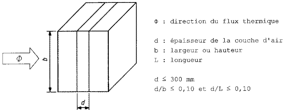
Figure [1] : Couche d'air ordinaire
