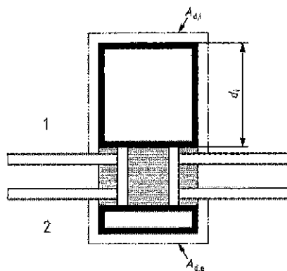
Figure [38] : Profondeur intérieure des traverses
