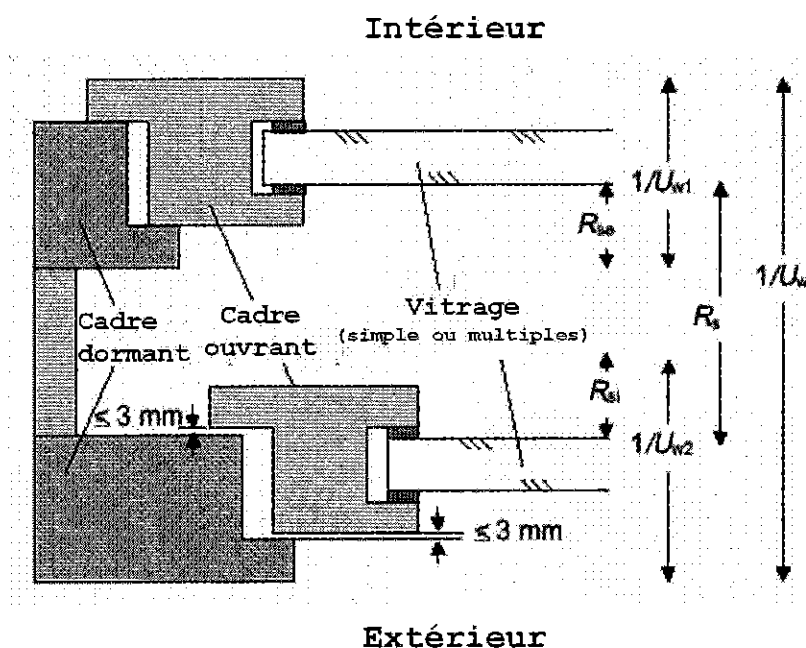
Figure [16] : Illustration d'une double fenêtre
