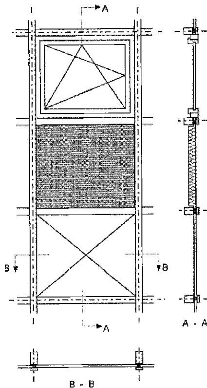
Figure [20] : Module d'une façade légère (mur rideau)
